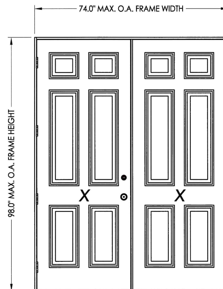
DOUBLE DOOR ELEVATION
