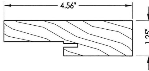
1 HEAD & SIDE JAMB
